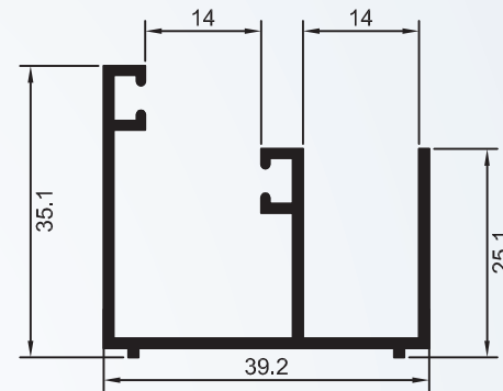
BX-141 2,690 Kg/BARRA 6m
