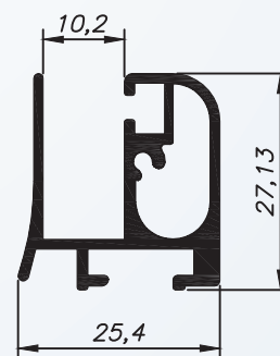
JP-084 2,910 Kg/BARRA 6m
