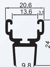
BX-133 1,716 kg/BARRA 6m
