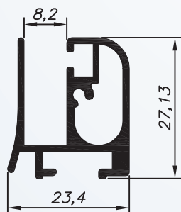
JP-083 2,970 Kg/BARRA 6m
