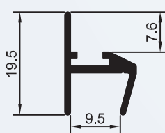
BX-131 0,900 Kg/BARRA 6m
