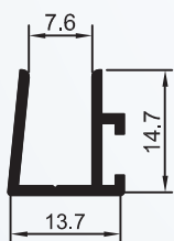
BX-128 0,850 Kg/BARRA 6m
