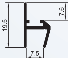
BX-130 0,800 Kg/BARRA 6m
