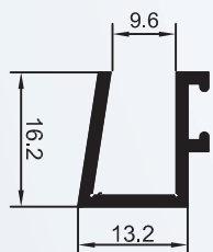
3172 0,850 Kg/BARRA 6m
