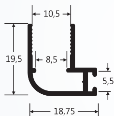
BX-251 1,070 Kg/BARRA 6m
