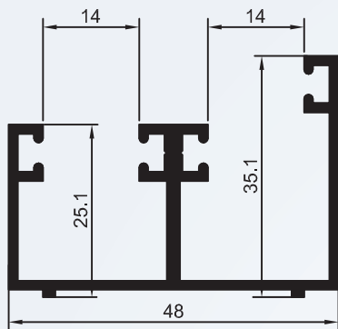
BX-150 3,900 Kg/BARRA 6m
