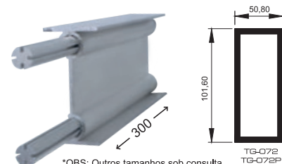
CHU 072-3 Chumbador Lm008 alumínio 300mm
